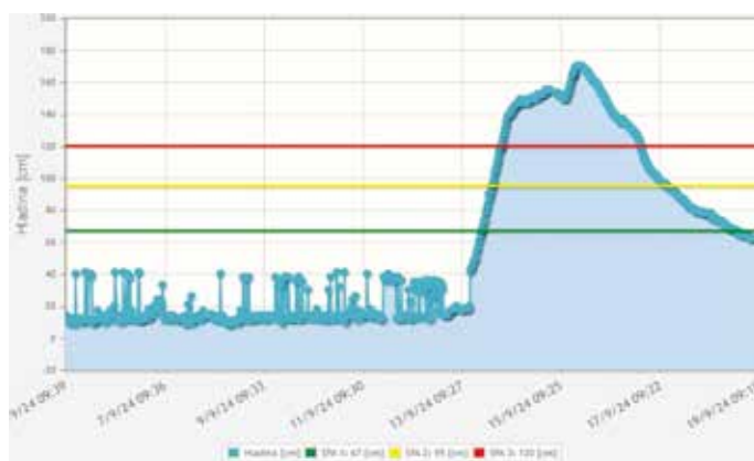
Vývoj stavu povodňové aktivity toku Romže - Držovice
