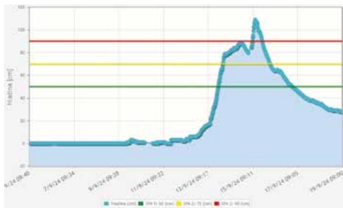
Vývoj stavu povodňové aktivity toku Romže - Stražisko
